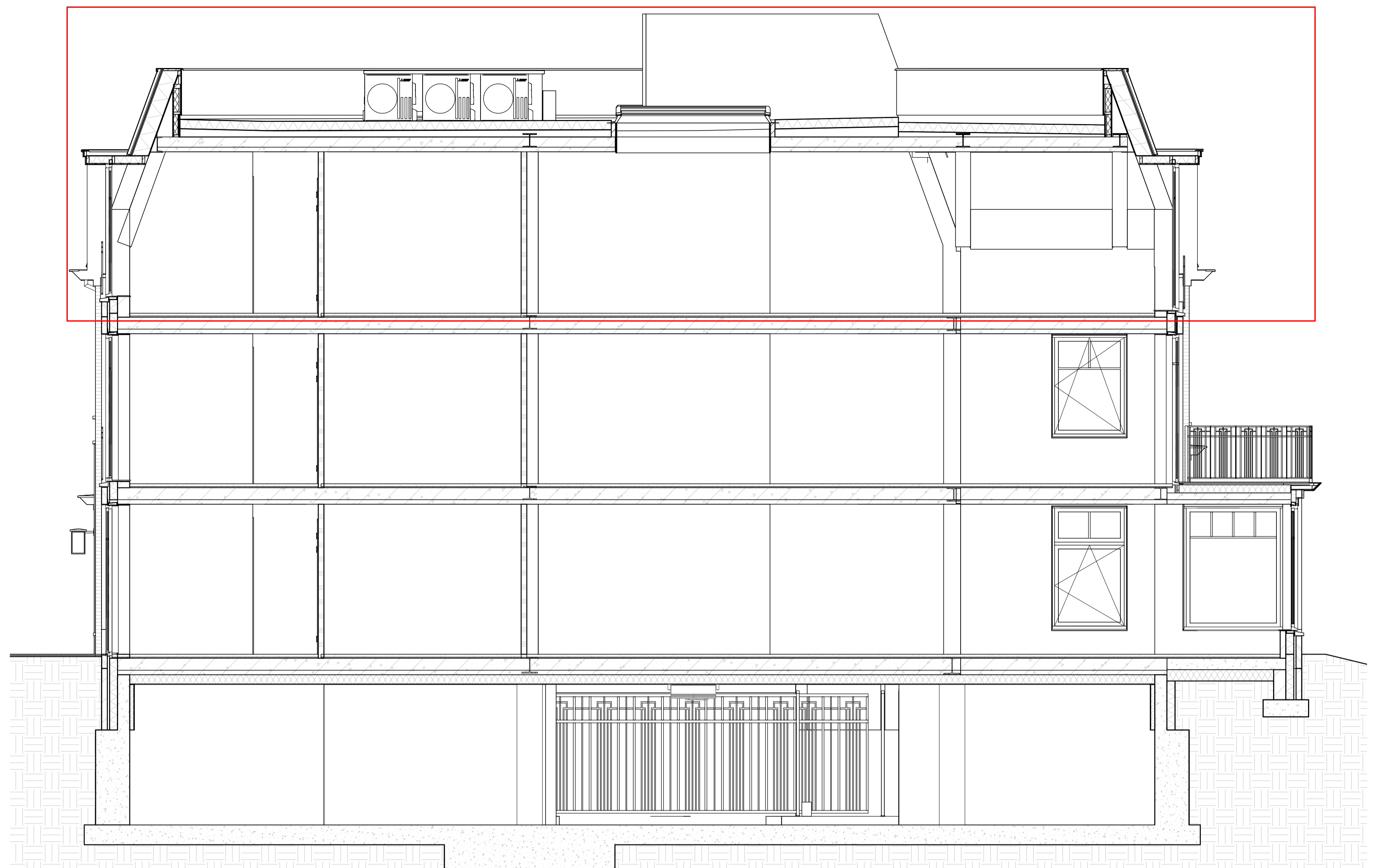
Doorsnede A
