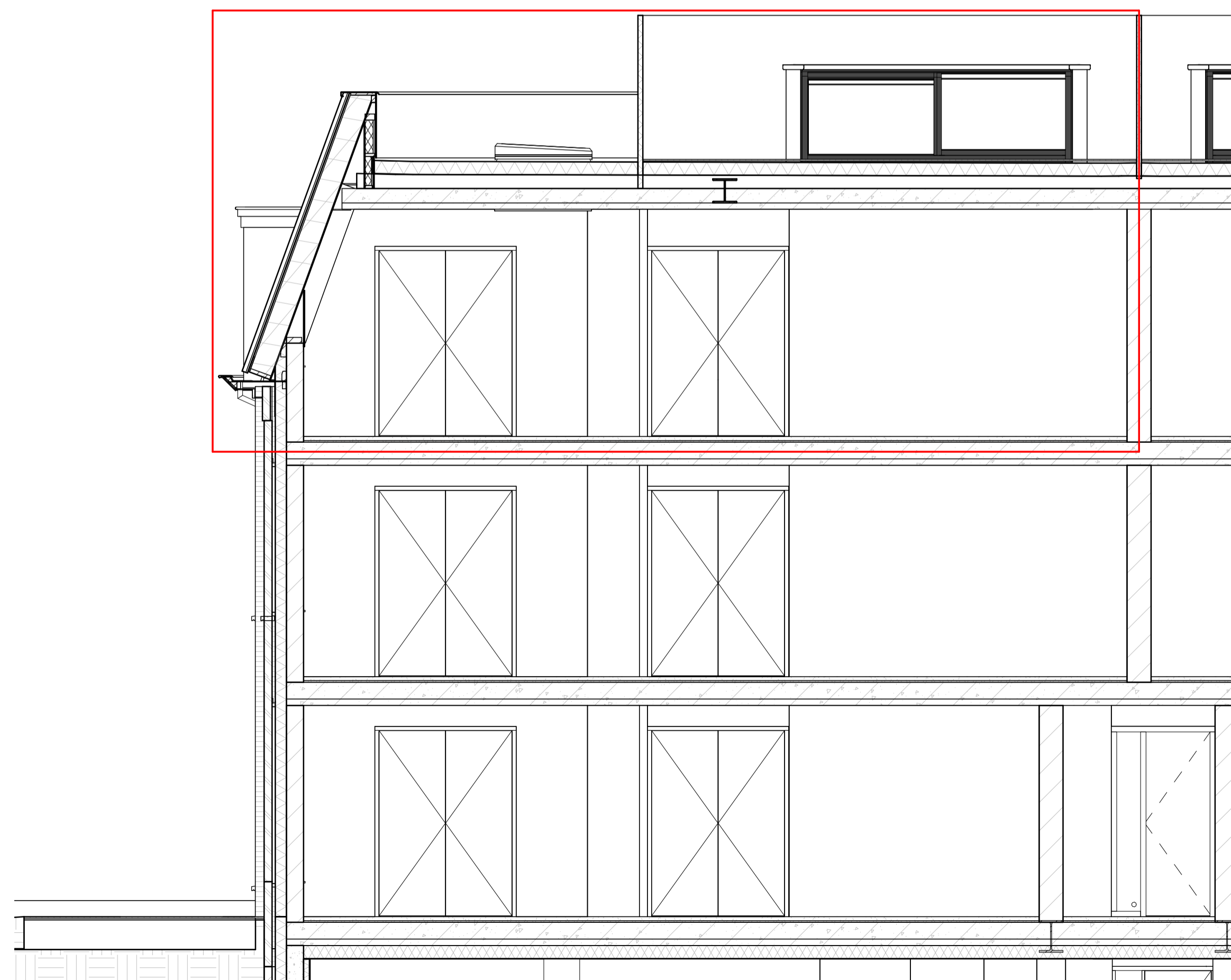
Doorsnede B
